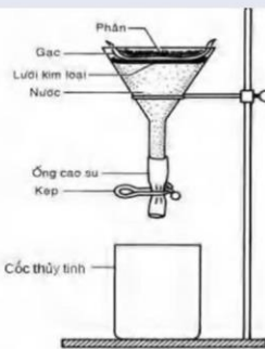
Hình 6.3. Hệ thống dụng cụ lọc (Nguồn Practical guide to Diagnostic Parasitology, Lyne S. Garcia)
