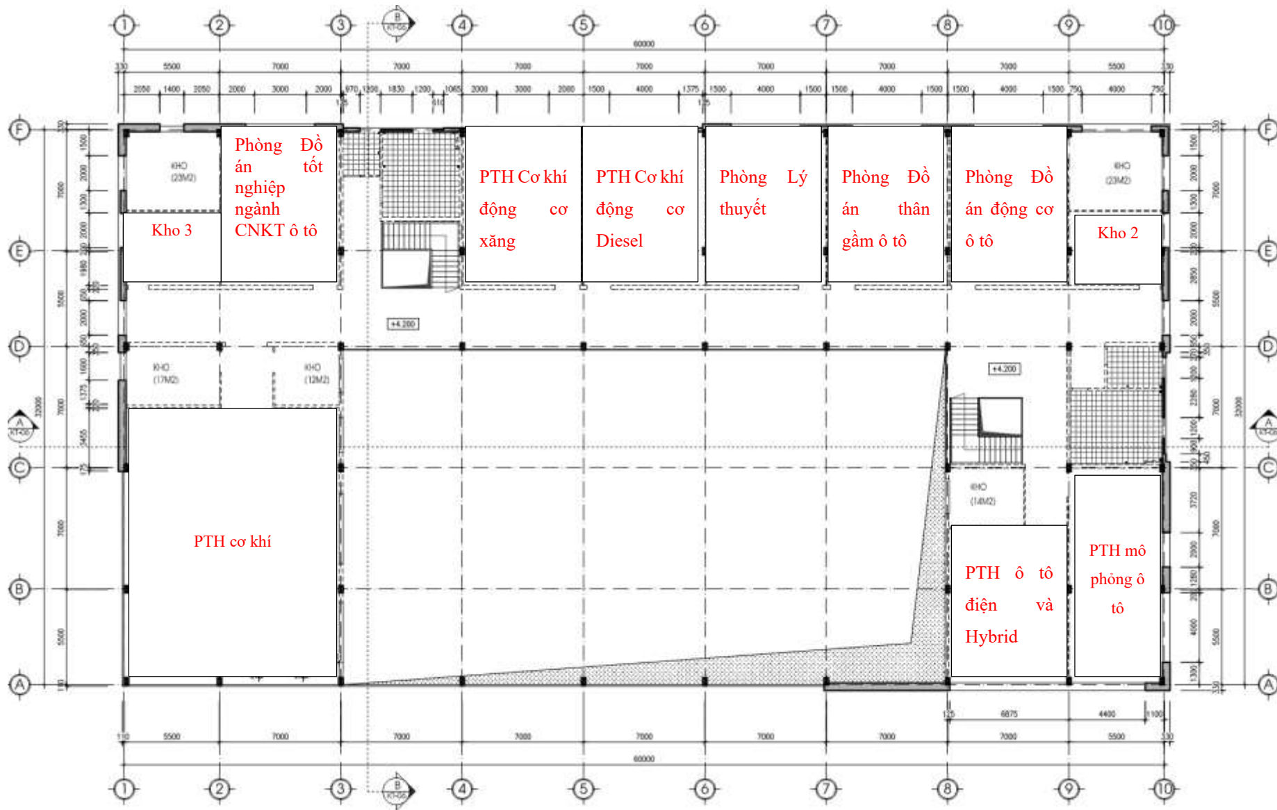
MẶT BẰNG BỐ TRÍ THIẾT BỊ, CẦU NẰNG TẦNG 2
