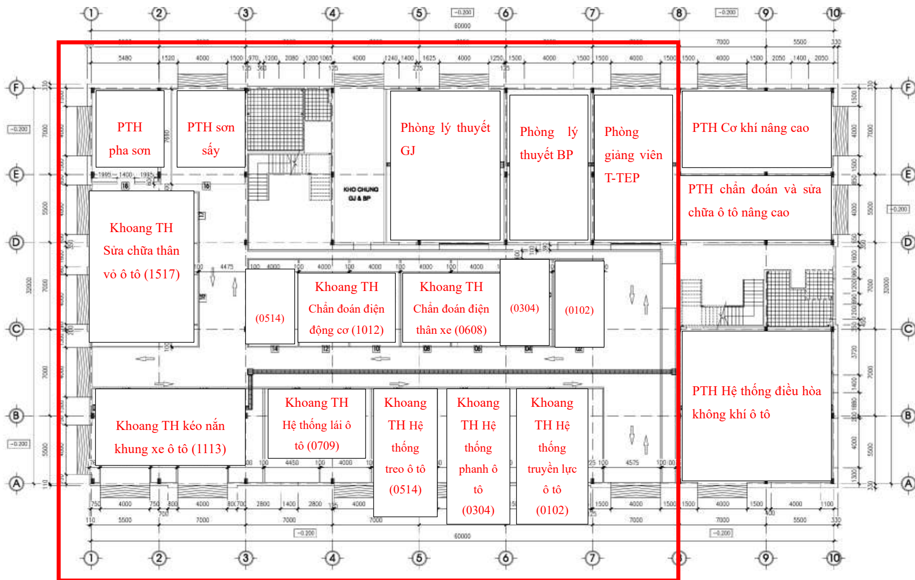
MẶT BẰNG ĐÁNH SỐ KHOANG LÀM VIỆC
